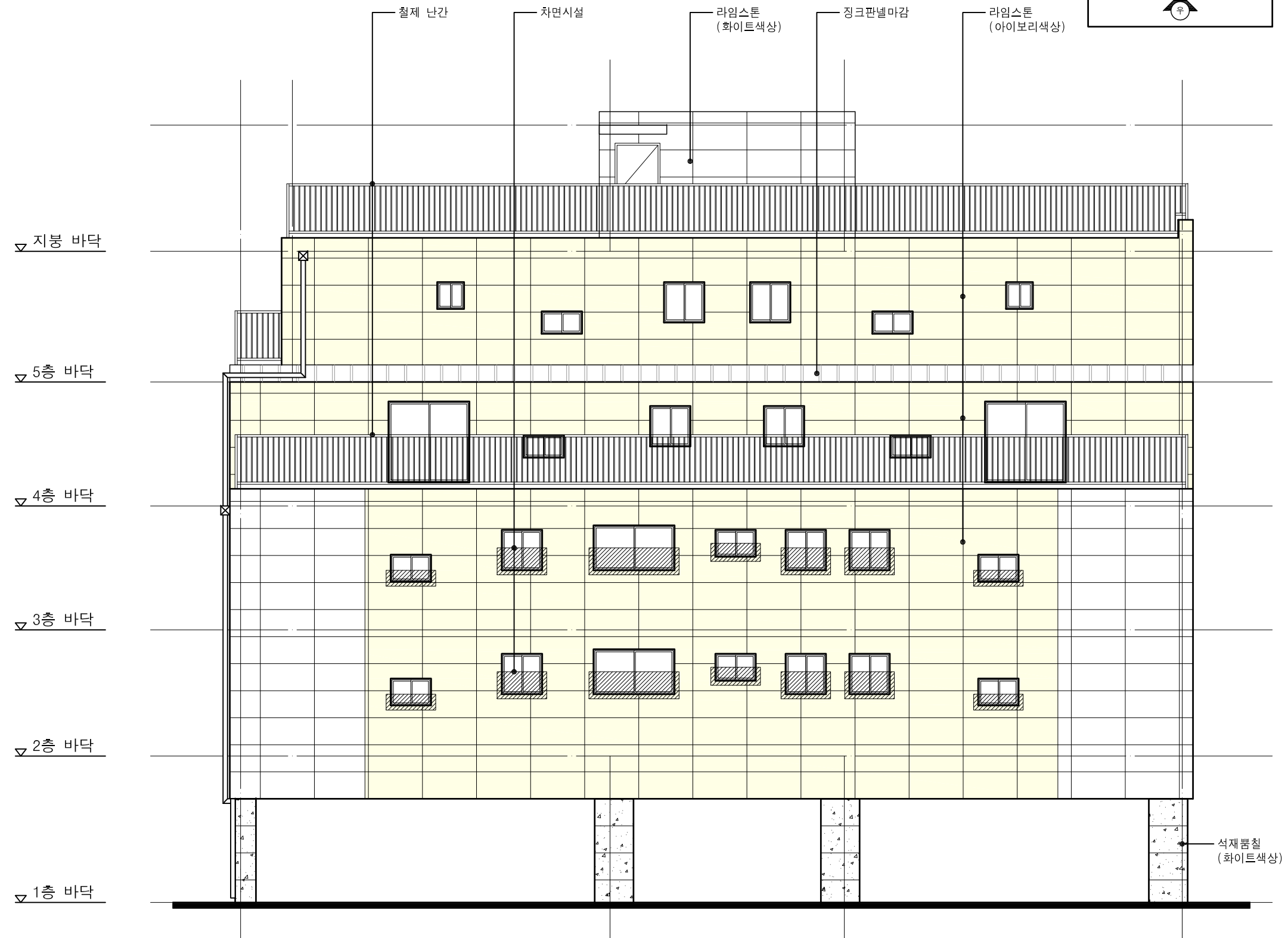
좌측면도 SCALE : A3 : 1/100
