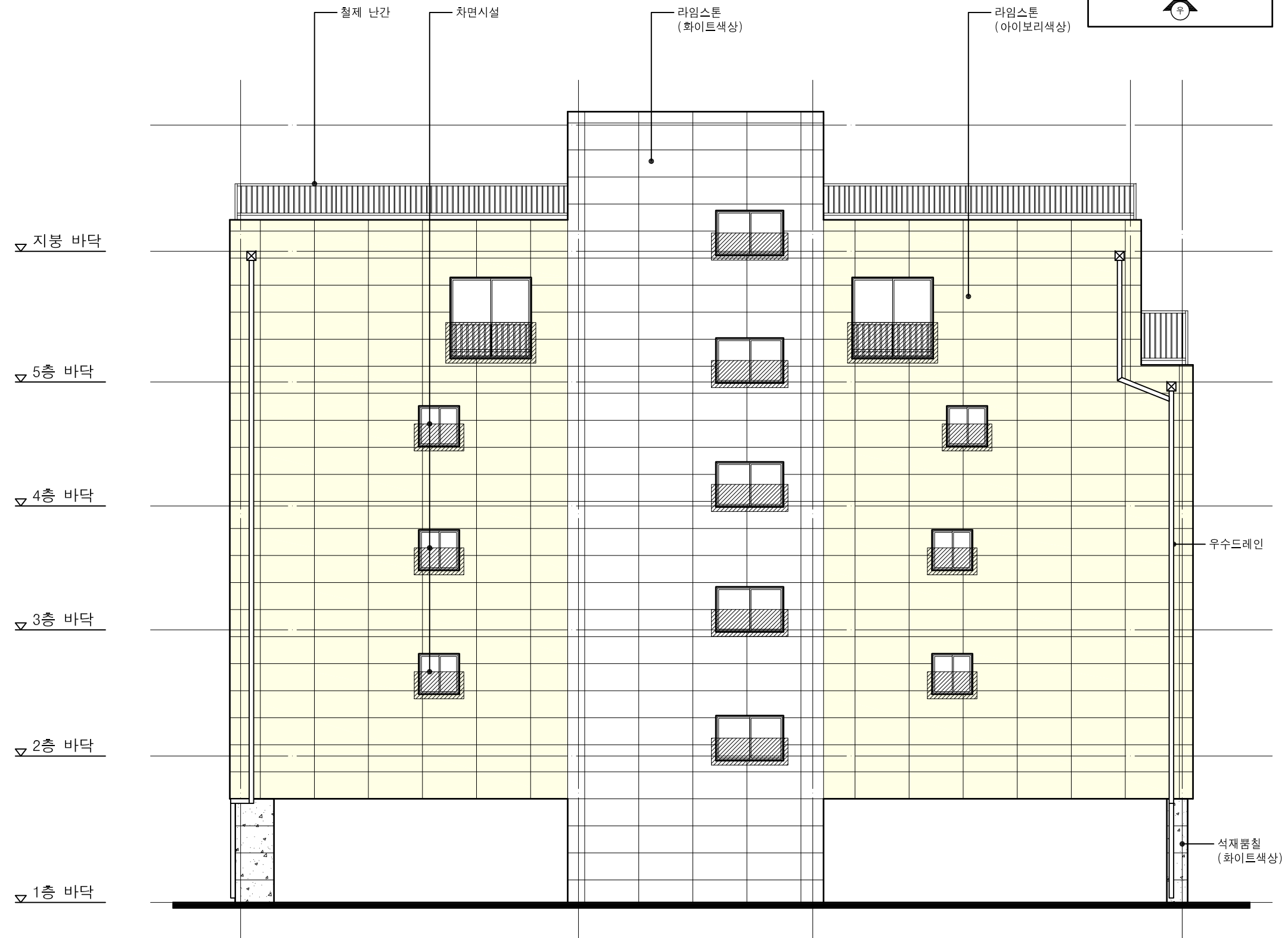
우 측 면 도 SCALE : A3 : 1/100
